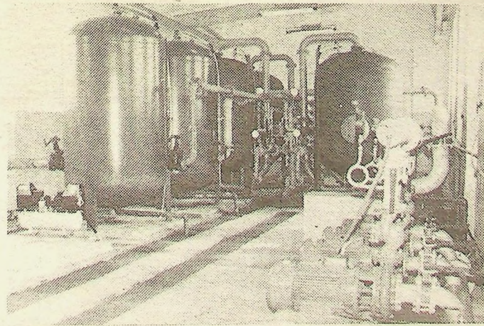
Stacja uzdatniania wody w Lisowicach.
