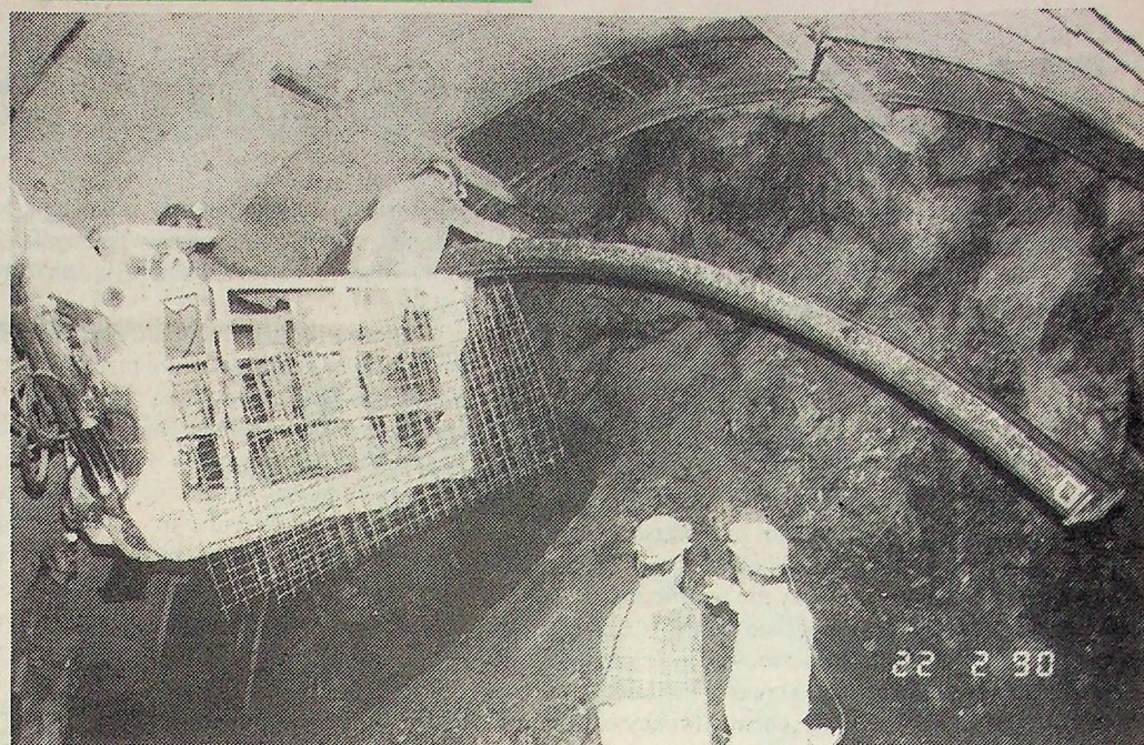
Montaż obudowy w tunelu Metsovo (Grecja).
