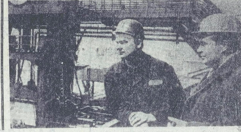
СВЕРДЛОВСКАЯ ОБЛАСТЬ. На Институтском местном комбинате имени Ленина начала работу первая очередь цеха широкополосных балок — блоннинг «1500». На блоннинг «1500» будут прокатывать слэбы весом до 22 тонн. На снимке: оператор стана В. С. КУЛЯГИН знакомит инженера с «Азостали» М. В. КОСАРЕВА с работой нового агрегата. Фото А. Грахова. (Фотохроника ТАСС).
