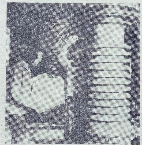
Высокоточные изоляторы фарфоровой фабрики города Печ (ВНР) установлены на действующей линии электропередачи, связывающей республику с советским городом Мукачевом. Они будут установлены и на проектируемой ЛЭП-750, по которой энергия пойдет в Венгрию из СССР.
