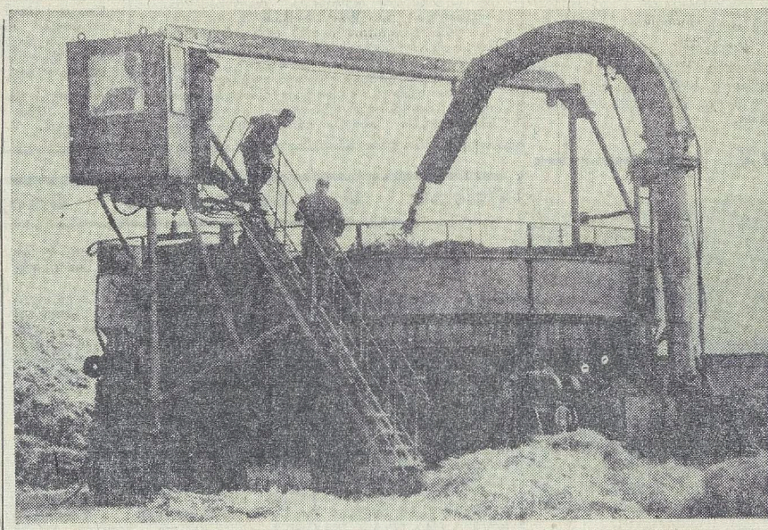
ВОРОНЕЖСКАЯ ОБЛАСТЬ. Два трехсоттонных циндарических стога свекловичной ботвы на силос недавно заготовили в колхозе «Великий Октябрь» Хохловского района с помощью пресс-машин «АВС-40». Ее сконструировал воронежский инженер Р. Т. Васильев. С помощью новой машины можно закладывать на силос или сенаж зеленую массу кукурузы, свекловичную ботву, соломенную резку.
