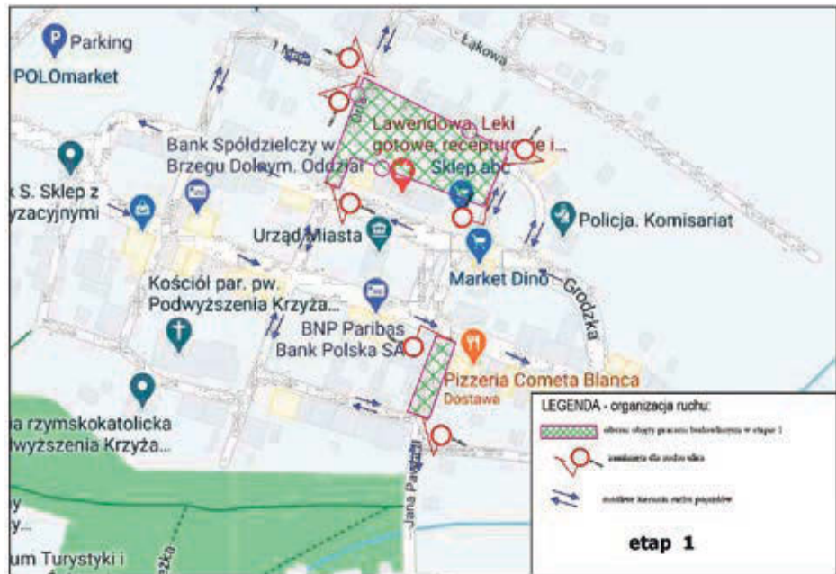
Schemat organizacji ruchu, obowiązujący na czas prowadzenia robót budowlanych w ramach etapu 1 rewitalizacji nawierzchni w centrum Ścinawy, czyli w obrębie ulic: Orlej i 1 Maja
