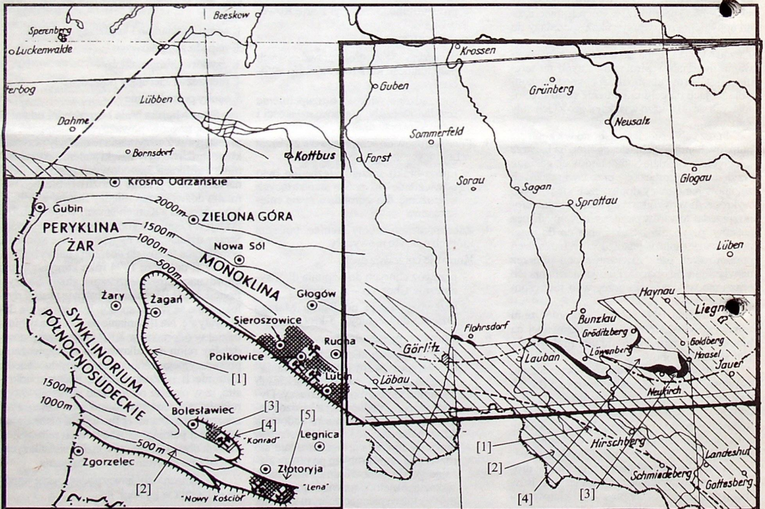
Rys. 2. Występowanie cechsztynu i złóż miedzi na Dolnym Śląsku według Jana Wyzykowskiego. Na podstawie pracy: Surowce mineralne Dolnego Śląska (praca zbiorowa). Wyd. Zakład Narodowy im. Ossolińskich PAN (Wrocław, Warszawa, Kraków, Gdańsk – 1979 rok)
