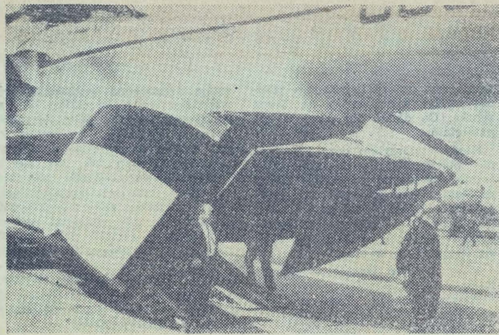
MI-6 (foto nr 1). P. latarnia mleczna w swej ladowni samochod ciężarowy lub traktor. Ciężar startowy - 42,5 tony; udźwieg eksploatacyjny - 12 ton. Zasięg lotu - 1050 km, szybkość 300 km/godz.
