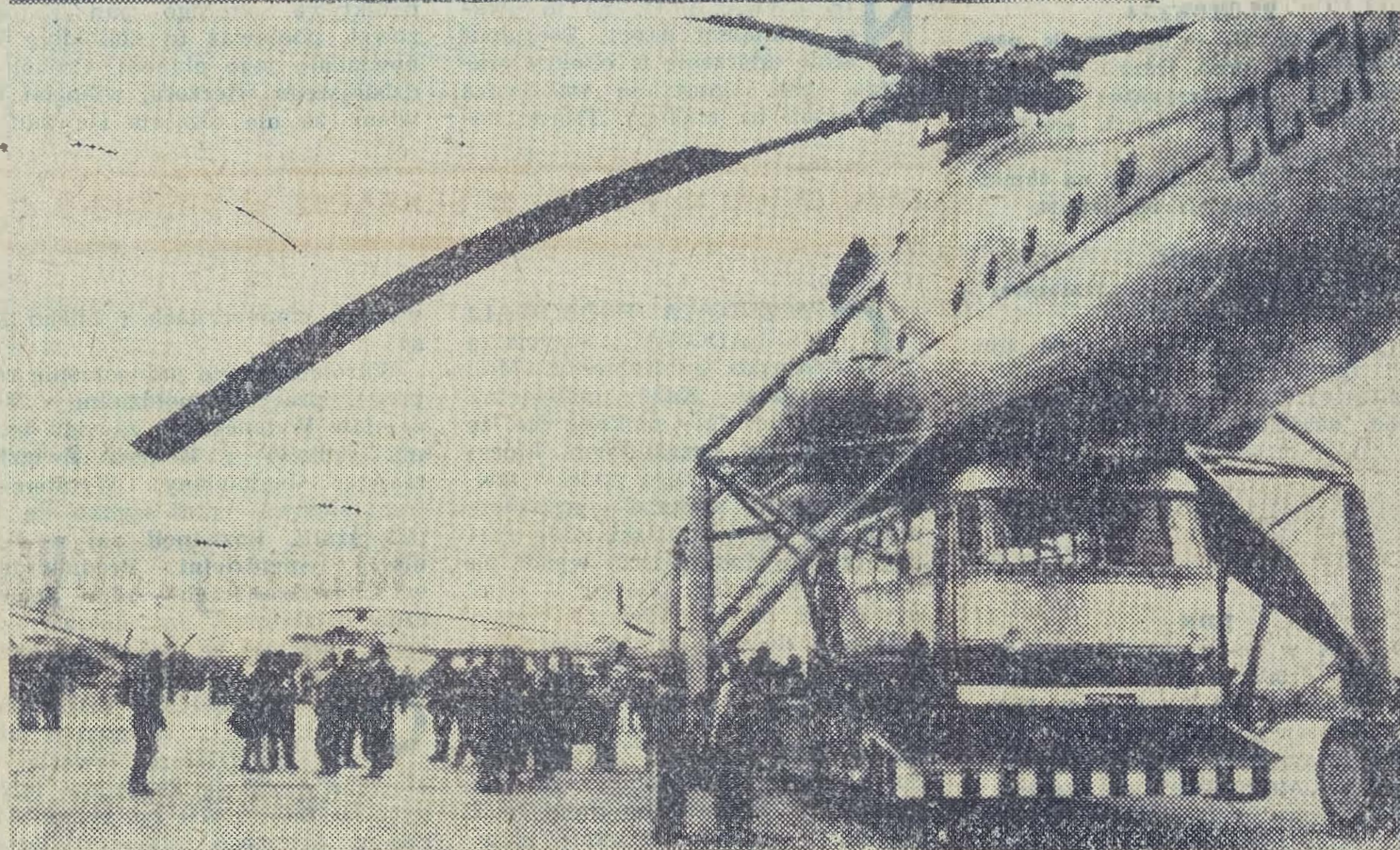
MI-10 (foto nr 3). Ten bezłotkowy śmigłowiec unosi na specjalnej platformie autobus ciężarowy. Ciężar startowy 43 tony, udźwieg
