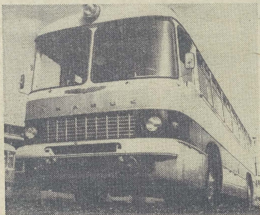
Budapeszteńska fabryka autobusów „Ikarus” rozpoczęła seryjną produkcję nowego autobusu dalekobieżnego „Ikarus-557”. Nowy autobus wyposażony jest w silnik umieszczony pod podłogą, odchylane fotele typu lotniczego i klimatyzację.
