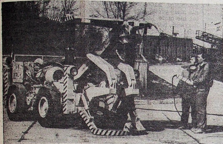
J. Miluch (z lewej) i R. Korga przy prototypie kotwiar ki prostowodowej. Fot. Cz. Baka
