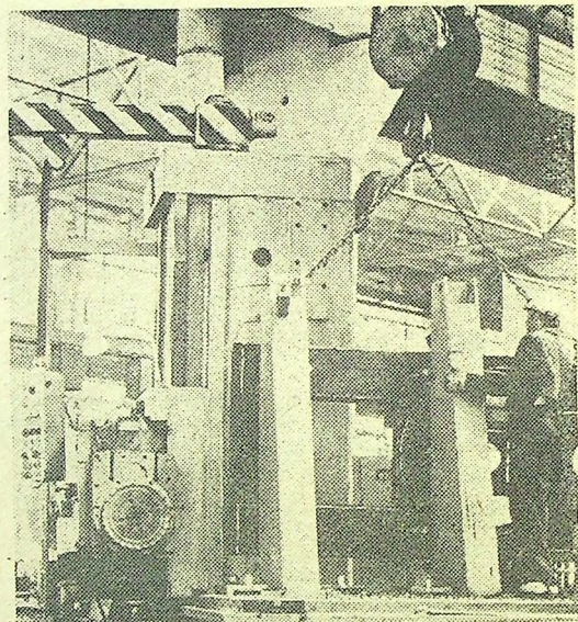
Wacław Suszek podczas wytaczania płyty płaskiej do żurawia typu „Hydros” K-1C2
