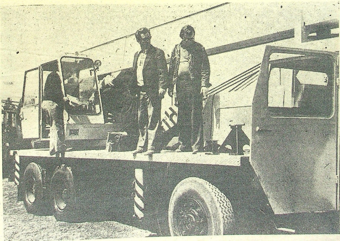
Przedstawiciele Przedsiębiorstwa Robót Zmechanizowanych Budownictwa Przemysłowego „Zachód” we Wrocławiu dokonują na placu fabrycznym przeglądu zakupionego „Hydrosa” 16T.
