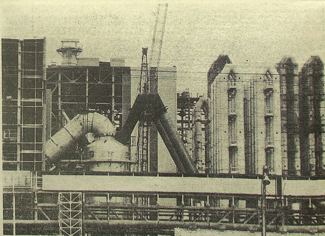
Tak wygląda kompleks Wydziału Metalurgicznego HM „Głogów 2”.
