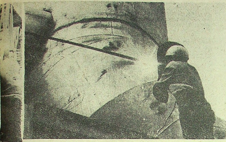
Spawacze niebawem zakończą swoją pracę. Czekają już na nich inne fabryki. Czesław Bleński spawa wymiennik ciepła E-208.
