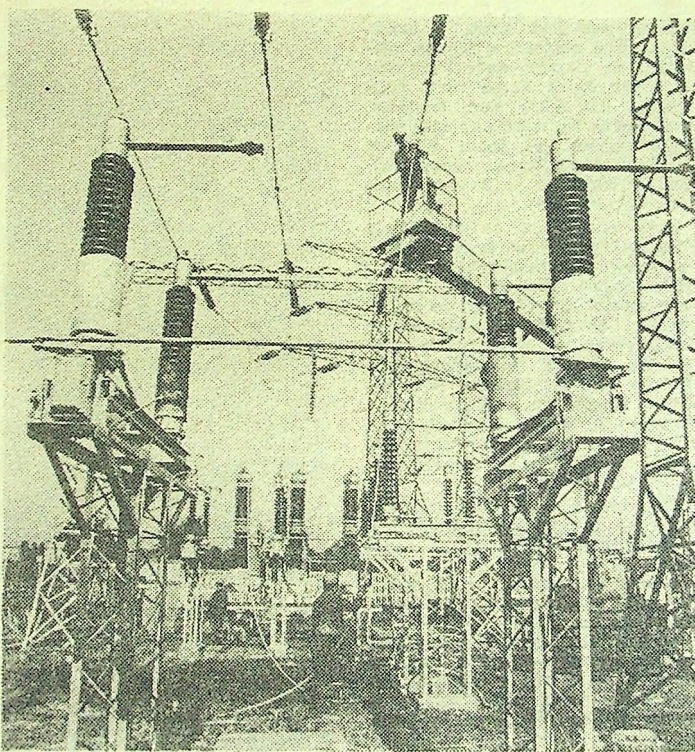
Ekipy katowickiego „Elbudu” przybyły do Legnicy 12 sierpnia i rozpoczęły prawie od podstaw odbudowę stacji przesyłowej Legnica-Północ.
