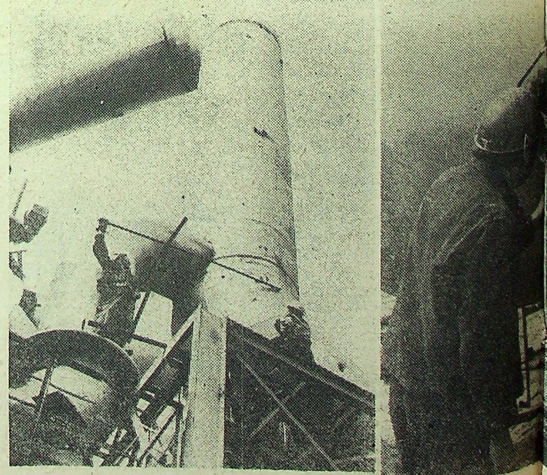
Większość prac wykonuje się na dużych wysokościach. Eugeniusz Stokłosa i Piotr Michalski montują rusztowania dla spawaczy.
