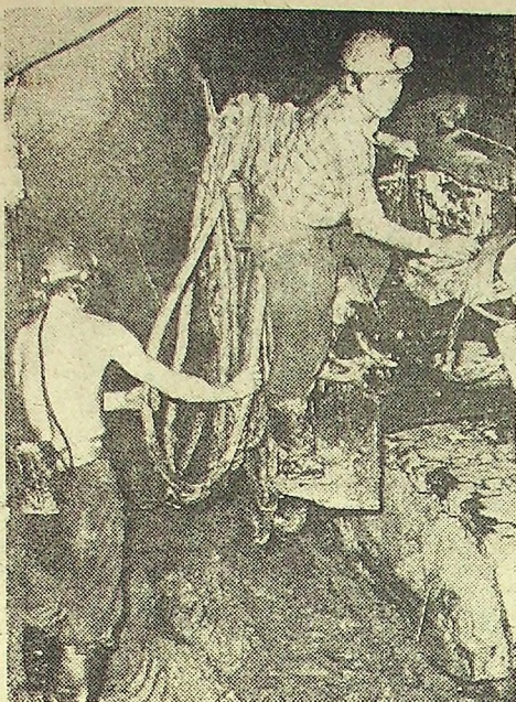
Operator ładowarki PNB-3K, Leszek Traj- kowski, wycofuje swoją maszynę z przodka.
