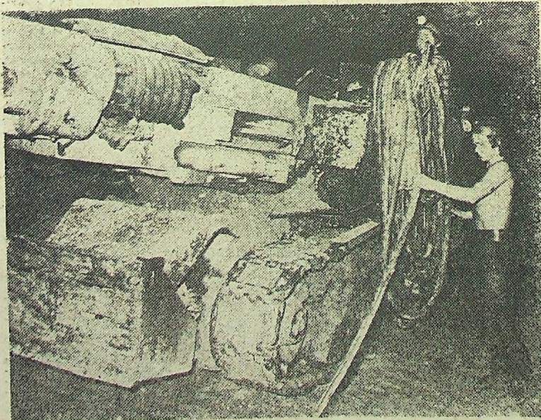
Podjazd na nowy przodek. Pomoceńnik Adam Bresso w trakcie układania kabli.
