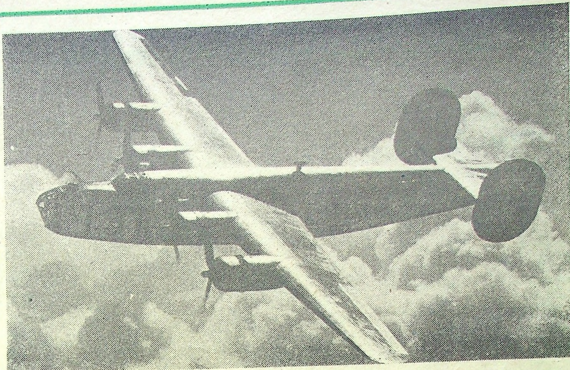
Samolot bombowy typu B-24 „Liberator” podczas lotu bojowego. Niektóre dane techniczne bombowca: rozpiętość skrzydeł — 33,5 m, długość — 20,5 m, uzbrojenie — 8—12 działek, ciężar całkowity — 27 ton, prędkość maksymalna — 450 km/godz. Fot. ze zbiorów autora
