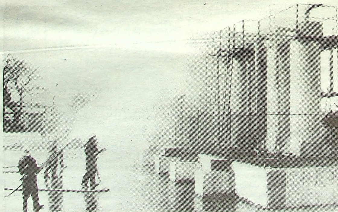
Schładzanie zbiorników z amoniakiem przed usunięciem awarii
