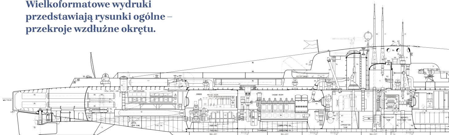
ORP ORZEŁ – RYSUNEK OGÓLNY – PRZEKRÓJ WZDŁUŻNY
